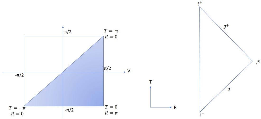
(a) Espace de Minkowski (bleu) dans les coordonnées (U, V) .
